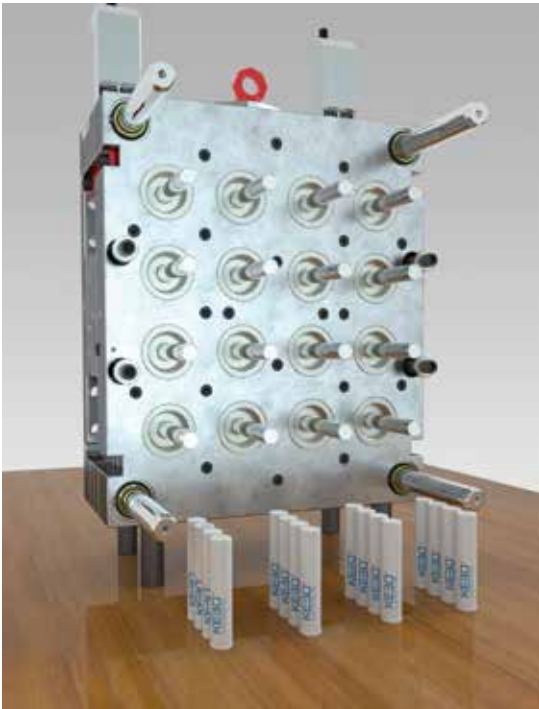
IML-Werkzeug, 16-fach Medizin
